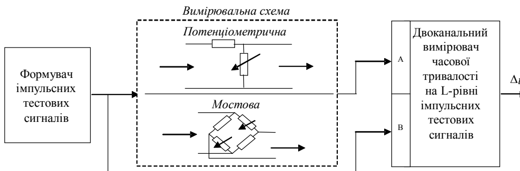
Рис. 3. Уніфікована структурна схема вимірювального каналу
